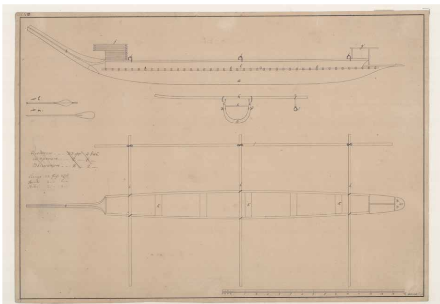
Figure 3.7. Ivan Koriukin, « Plan et dimensions d'une pirogue nukahivienne », encre. Bancroft Library , Université de Californie, Berkeley, 1963.002 : 1012.
